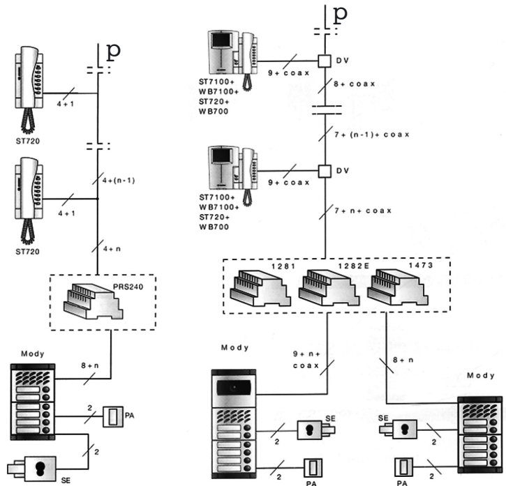
Exemple 1: Interphone de portail – conventionnel station.
