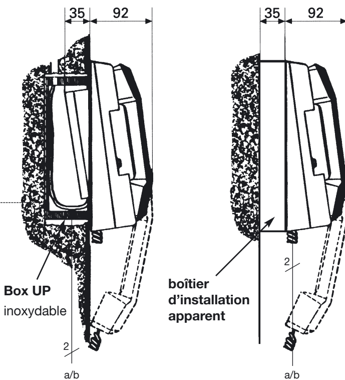
Montage encastré (UP) avec position d'attente
