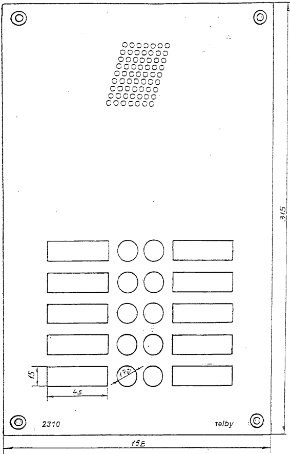
Freisprechtelefon telby 2310 mit 10 Rufasten für TVA- (Amt-) Anschluss Stahl geschliffen, 2,5 mm
