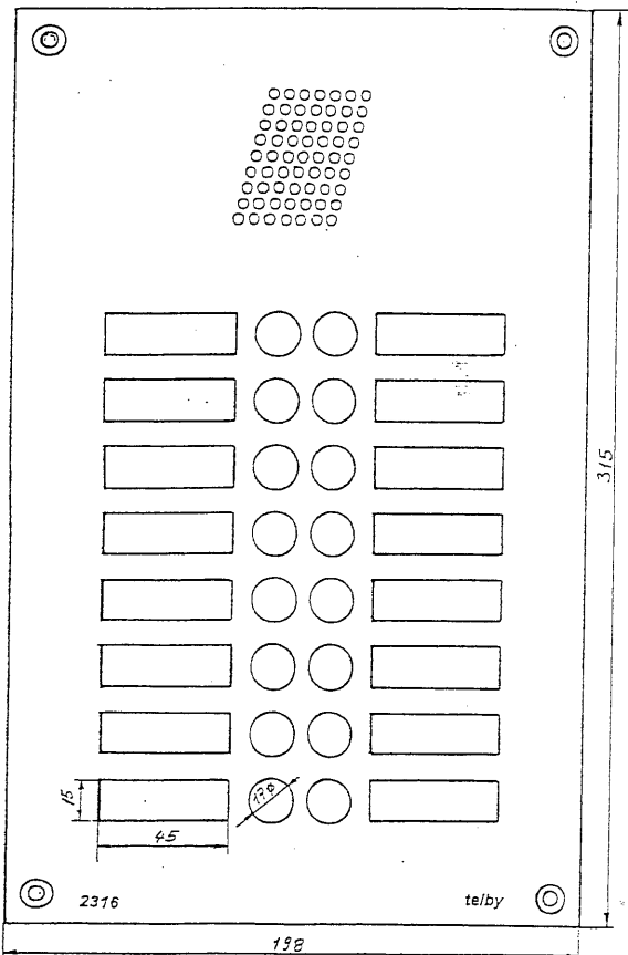
Freisprechtelefon telby 2316 (2318) mit 16 (18) Rufasten für TVA- (Amt-) Anschluss Stahl geschliffen, 2,5 mm
