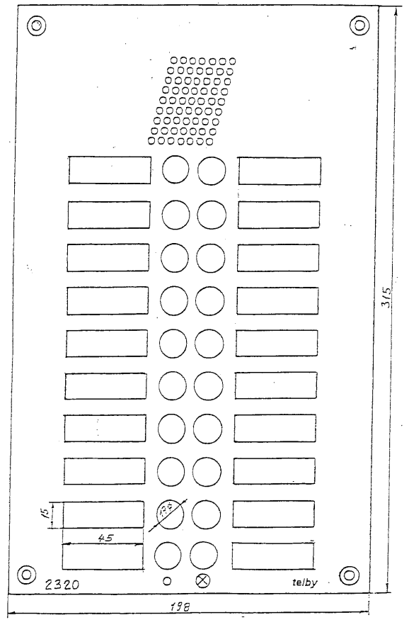
Freisprechtelefon telby 2320 mit 20 Rufasten für TVA- (Amt-) Anschluss Stahl geschliffen, 2,5 mm
