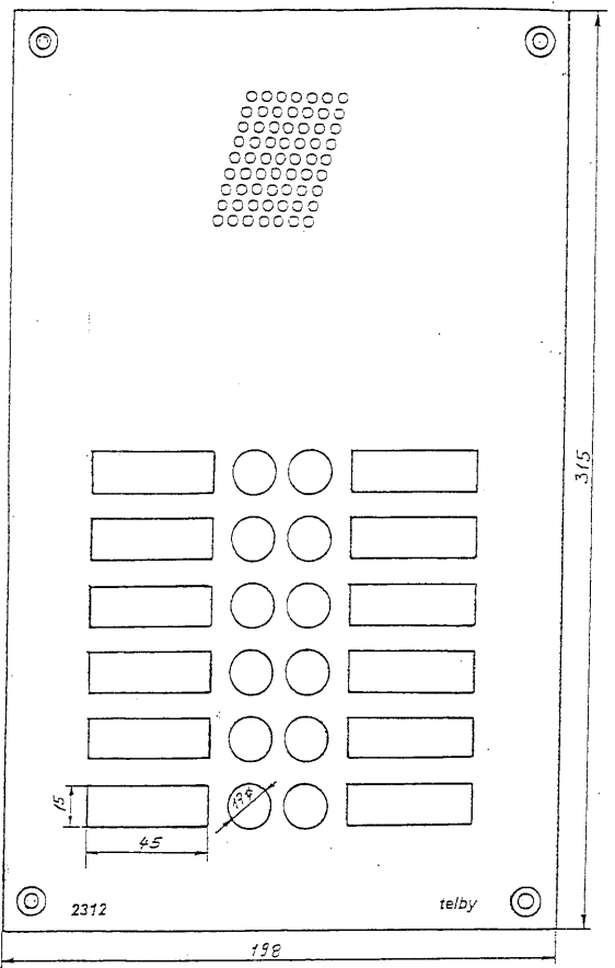
Freisprechtelefon telby 2312 (2314) mit 12 (14) Rufasten für TVA- (Amt-) Anschluss Stahl geschliffen, 2,5 mm
