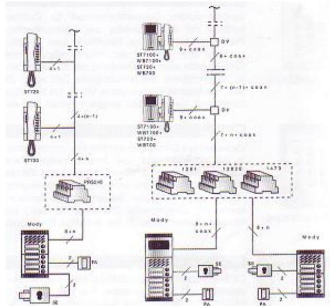
Beispiel 1: An eine Türstation ange- schlossene Haustelegone - konventionelle Anlagenart.
