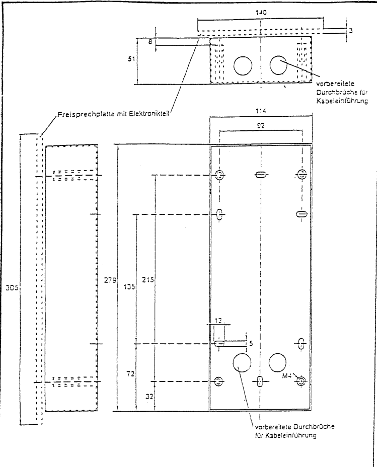
Wand-Einbaubox zu Freisprechtelefon telby RA 711 VANDAL RESIST
