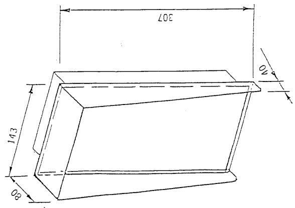
Regenschutzhäube für UP - Montage (hinter Frontplatte geklemmt)
