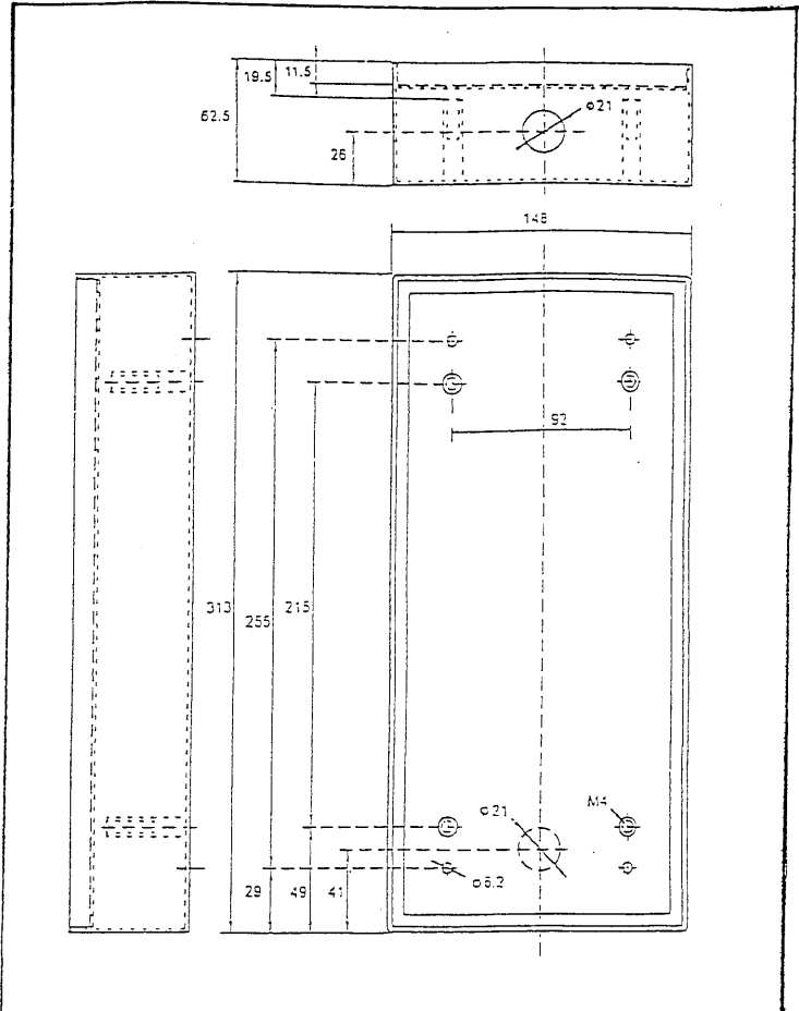
Surface-Box zu Freisprechtelefon telby RA 711 VANDAL RESIST Kabeleinführung von unten (oben) A11552 8D5 Kabeleinführung von hinten A11554 598
